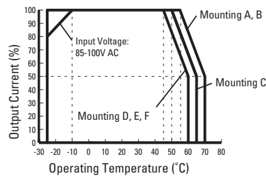
PS5R-VC24
