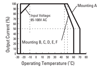
PS5R-VC12
