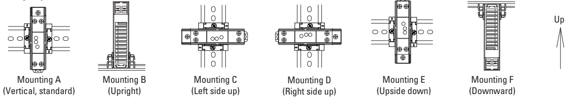
PS5R-VB/VC
