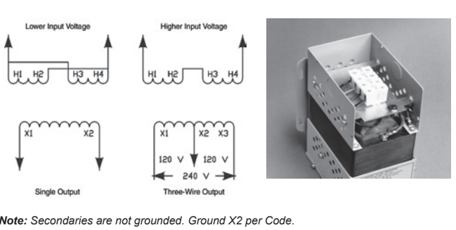
Figura 3. Conexiones Eléctricas para los Modelos No-8
