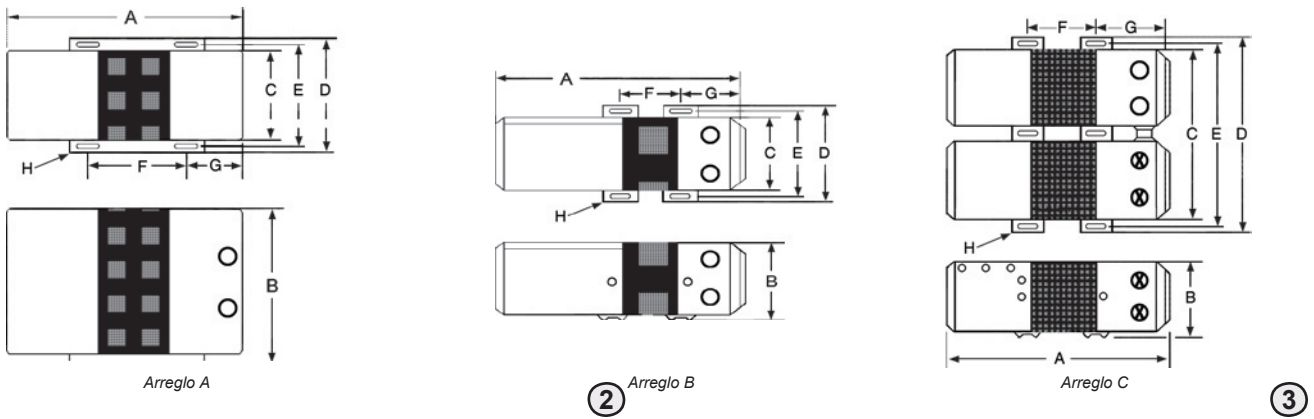
Figura 1: Agujeros de Montaje y Dimensiones
