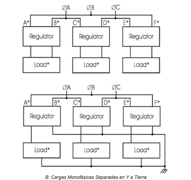
B: Cargas Monofásicas Separadas en Y a Tierra
