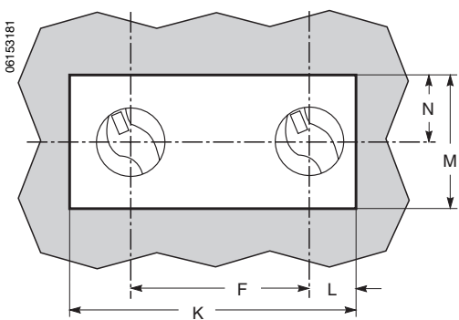
Front-panel Cutout
