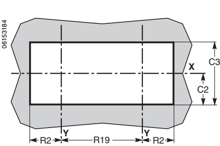
Front-panel Cutout
