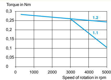
ILE1 without gearing
