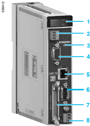
LMC 10
