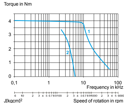
BRS39A
