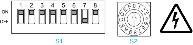
Parameter switches
