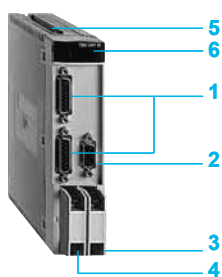
TSX CAY 21/22
