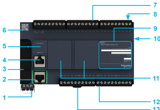
M221: 40 I/O
