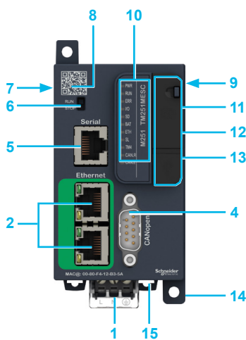
TM251MESD controller
