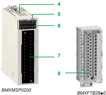
BMXFTB28●0
