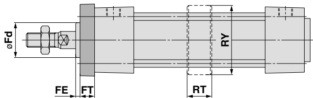
Rod Side Flange
