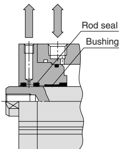
Relief port
