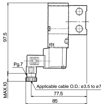
DIN terminal (D)
