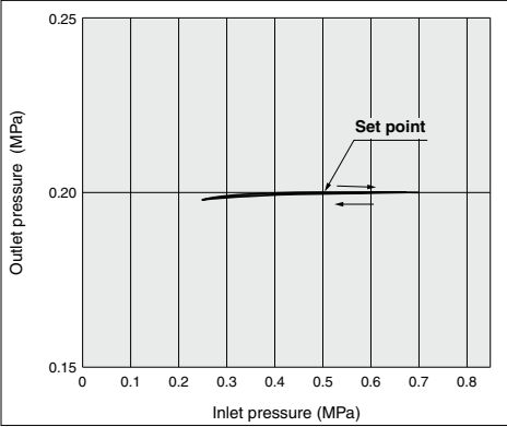
ARP30(K)
