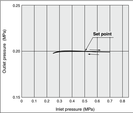
ARP20(K)
