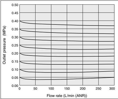
ARP20(K) Rc 1/4
