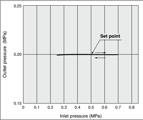
ARP40(K)
