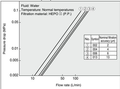
HEPO II element (P.P.): FQ1011N-06-R [Symbol]
