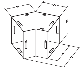
45° Elbow
