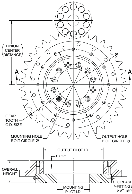
SECTION A-A
