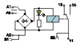
RB...121 AI
