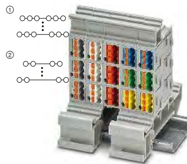
22 A, DIN rail mounting
