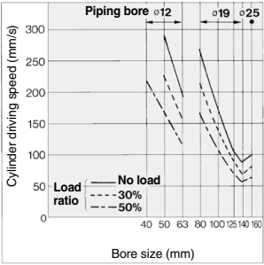
AS2000-01/02
