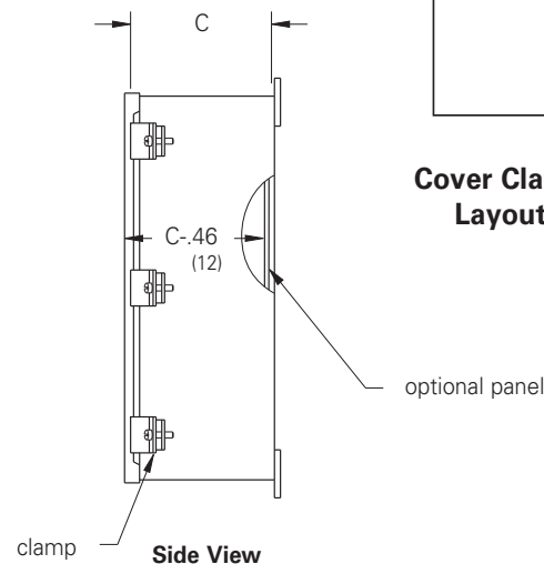
864-4XSCHC 884-4XSCHC 1084-4XSCHC 12106-4XSCHC 12126-4XSCHC 14126-4XSCHC 16146-4XSCHC
