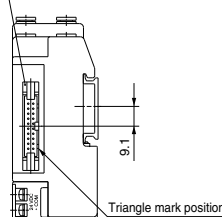
60PG (20 pins)
