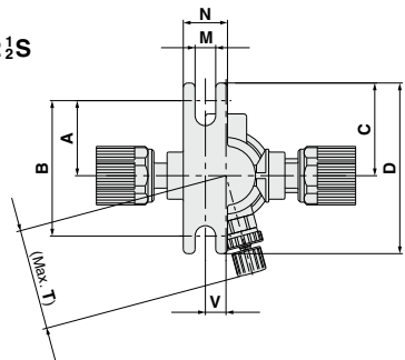
LVQ3 1 / 2 S, LVQ4 1 / 2 S LVQ5 1 / 2 S, LVQ6 1 / 2 S
