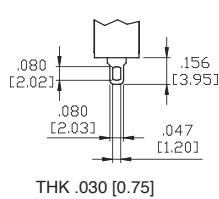
M1 Standard Solder Lug
