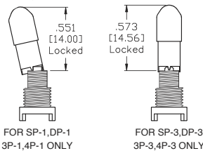
Locking Lever TI
