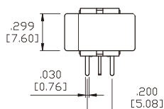
M6 Double Pole
