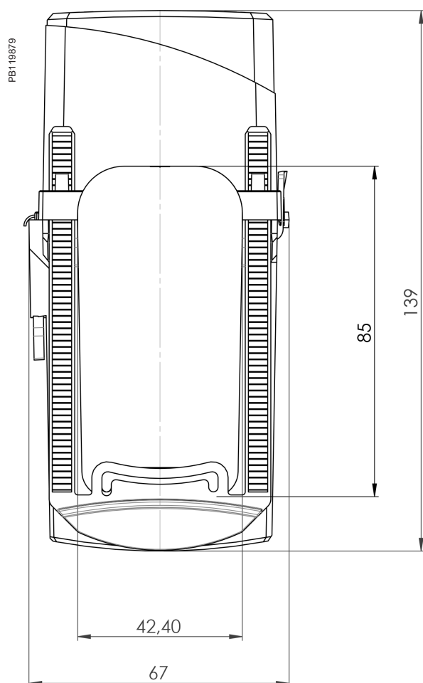
HM Dimensions
