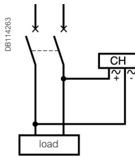
CH "48 x 48".
