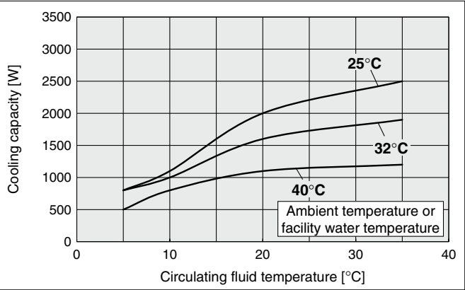
HRR030-A-20, HRR030-W-20
