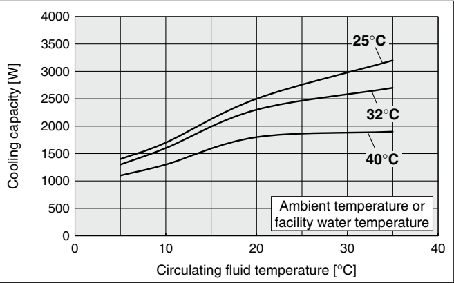
HRR050-A-20
