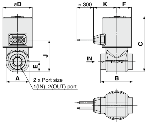
G: Grommet
