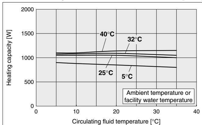
HRR050-A-20, HRR050-W-20
