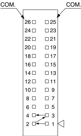
(P, PC: 26 pins)
