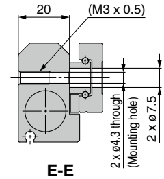
E-E
