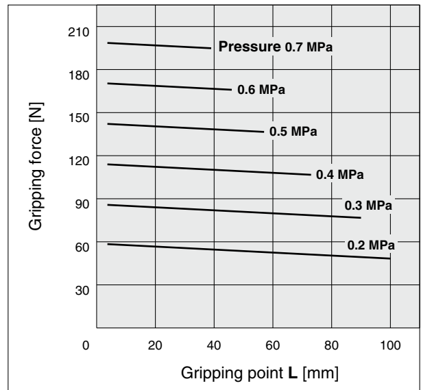
MHF2-20FD□
