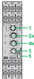
RM22UA3•MR
