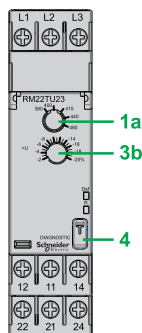
RM22TU
