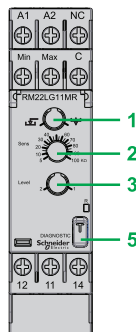
RM22LG11MR
