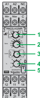
RM22LA32MR
