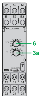
RM22JA21MR
