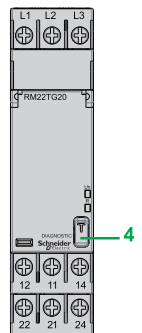
RM22TG
