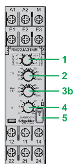
RM22JA31MR
