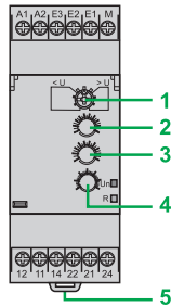
RM35 UA11MW/UA12MW/UA13MW
