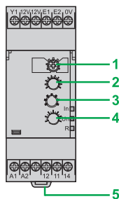
RM35S0MW
