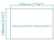
Cutout Dimensions
