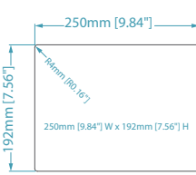
Cutout Dimensions
