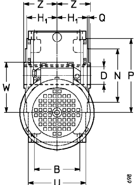
MR 2IV 100 ... 126
