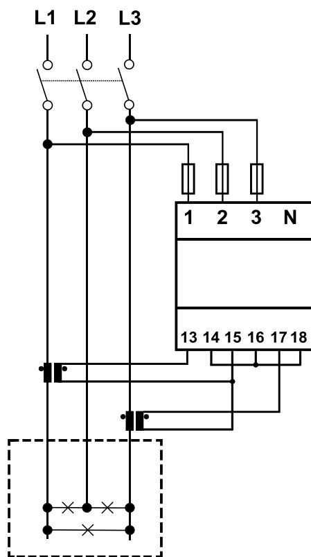
ARON trifásico (3 hilos)
